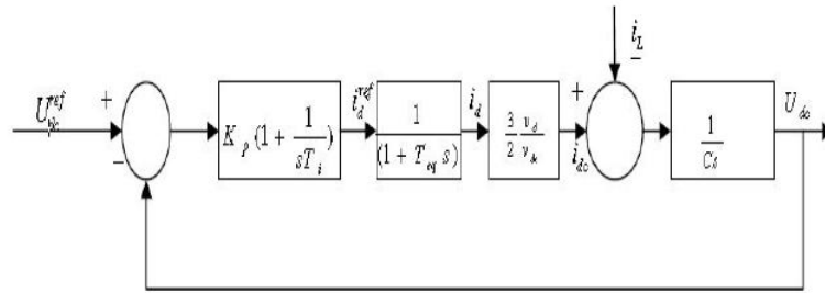
Fig 6. Dc voltage control loop in dq axes
