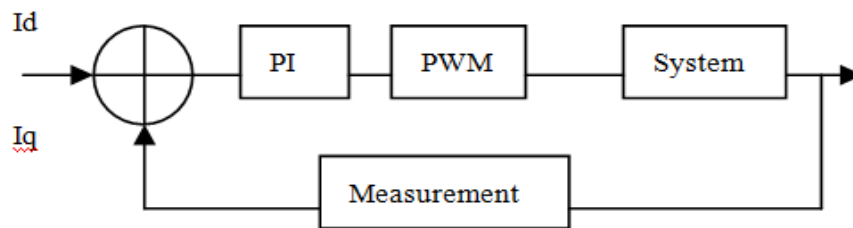
Fig. 4. The inner current control loop in dq axes.
